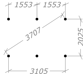
Runda plintar.
