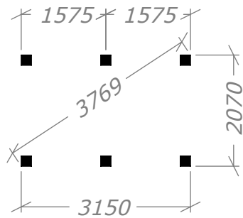
Fyrkantiga plintar.
